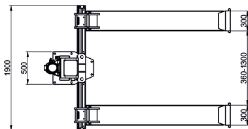
360mm mit optionalem Zubehör (Radgabeln)
