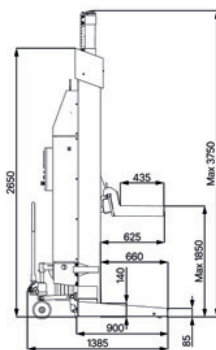
Beispielbild: 4 von maximal 16 Säulen
