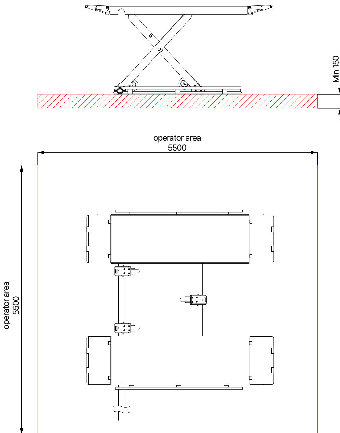
Σχέδιο θεμελίωσης επί εδάφους
