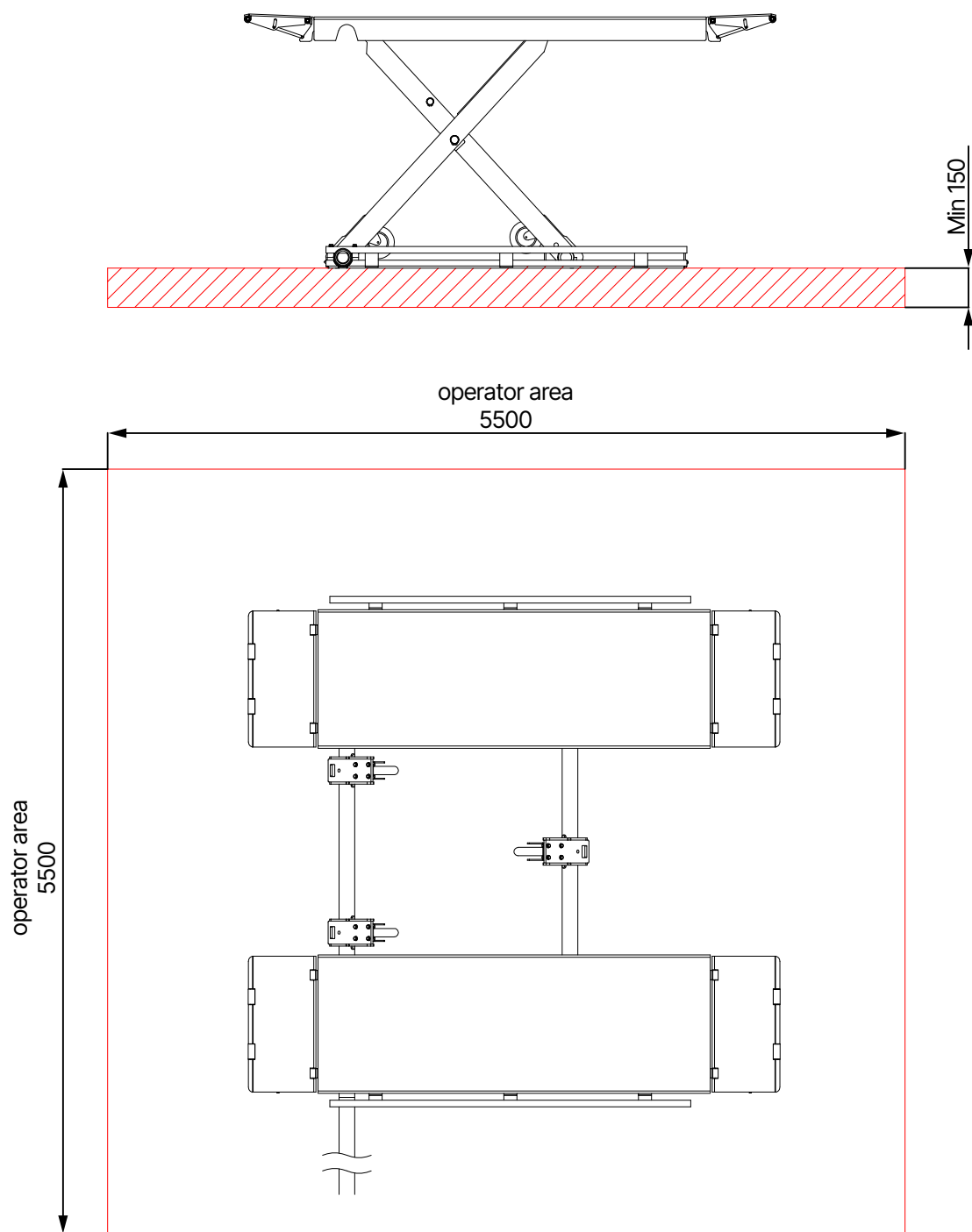
Půdorys nadzemních základů
