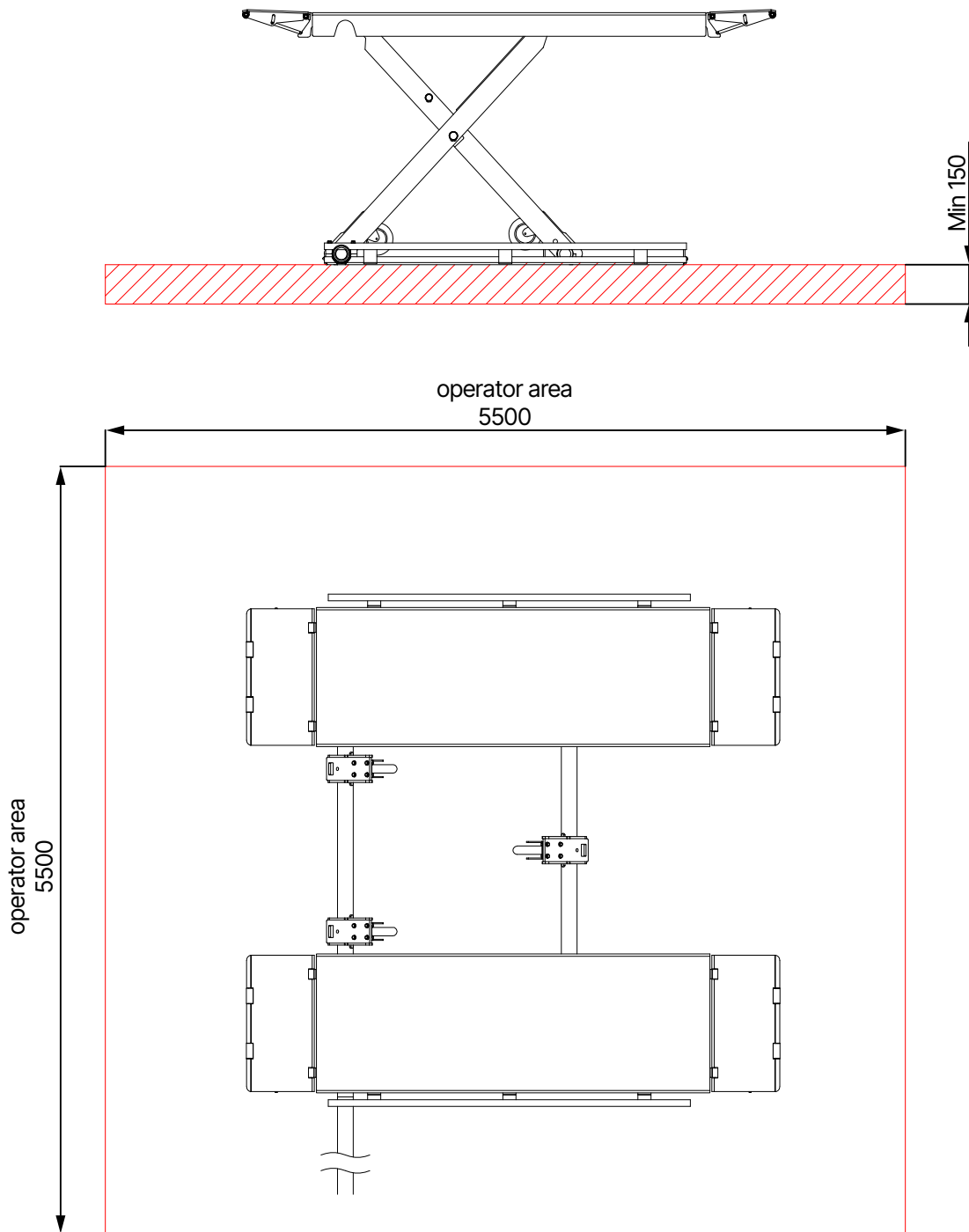
Fundamentplan Überflur
