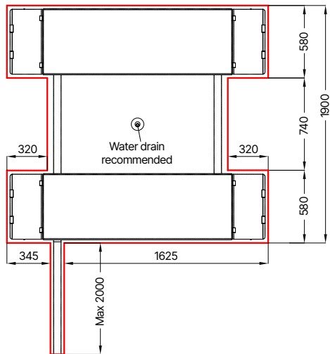
Funderingsplan ondergronds
