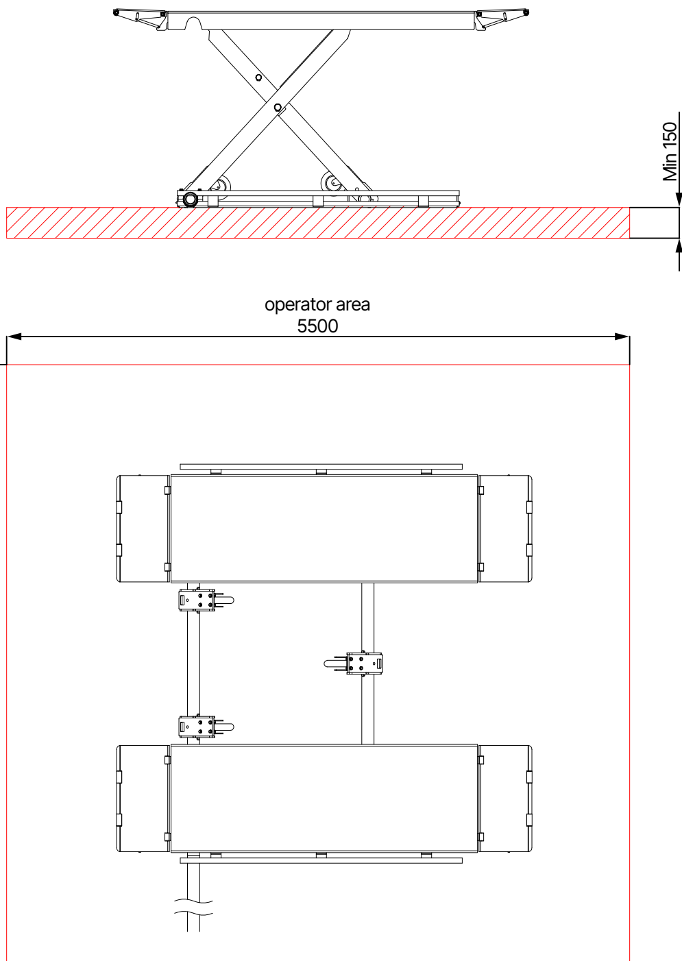
Maanpäällinen perustussuunnitelma
