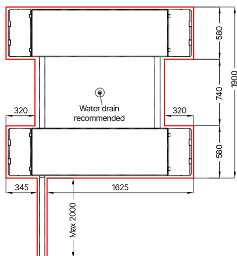
Základový plán pod podlahou
