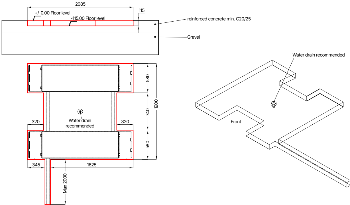
Σχέδιο θεμελίωσης κάτω από το δάπεδο
