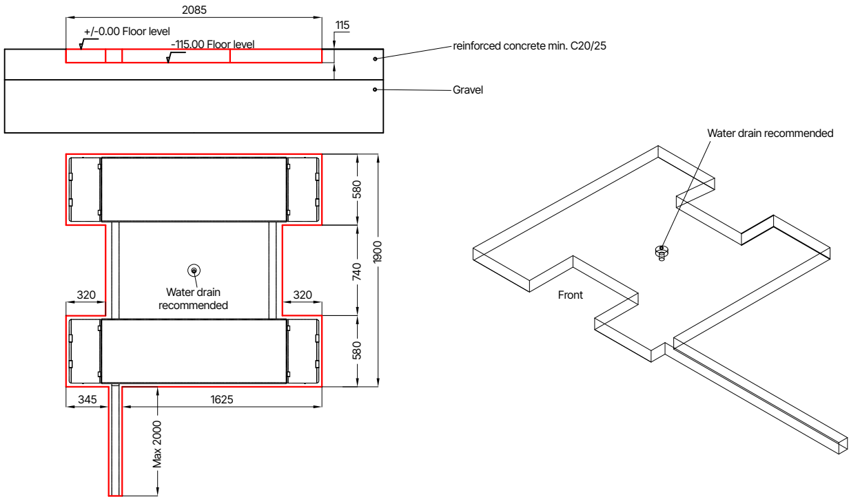
Plan de fondation sous le sol
