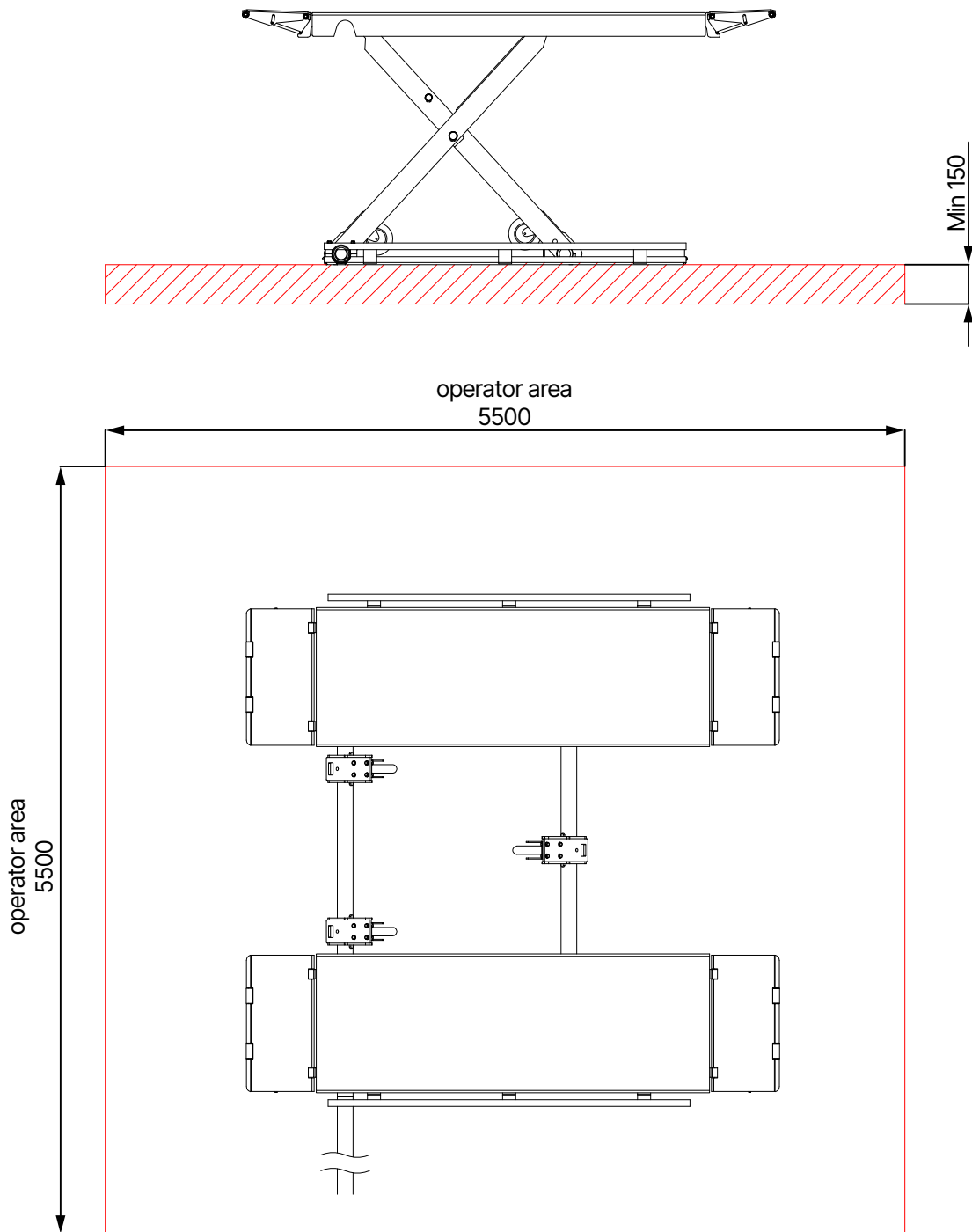
Funderingsplan bovengronds
