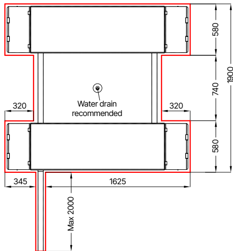
Plan fundamentów pod podłogą
