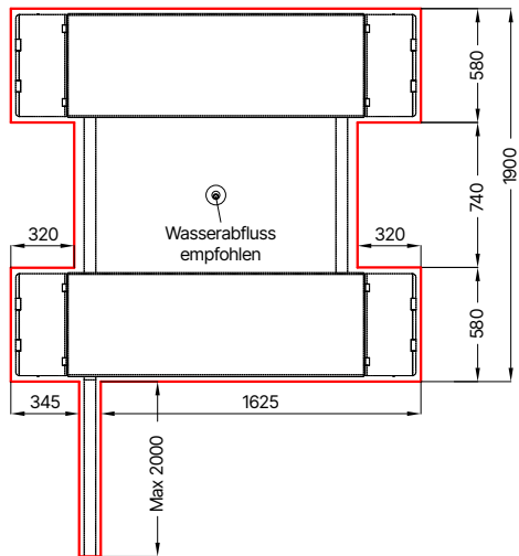
Fundamentplan Unterflur
