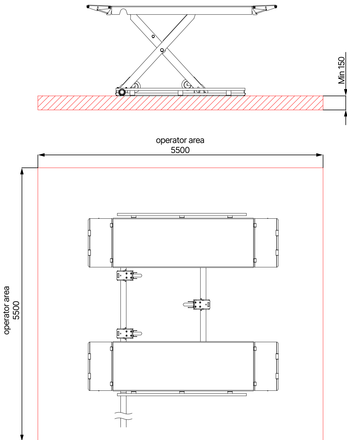
Plan de fondation hors sol
