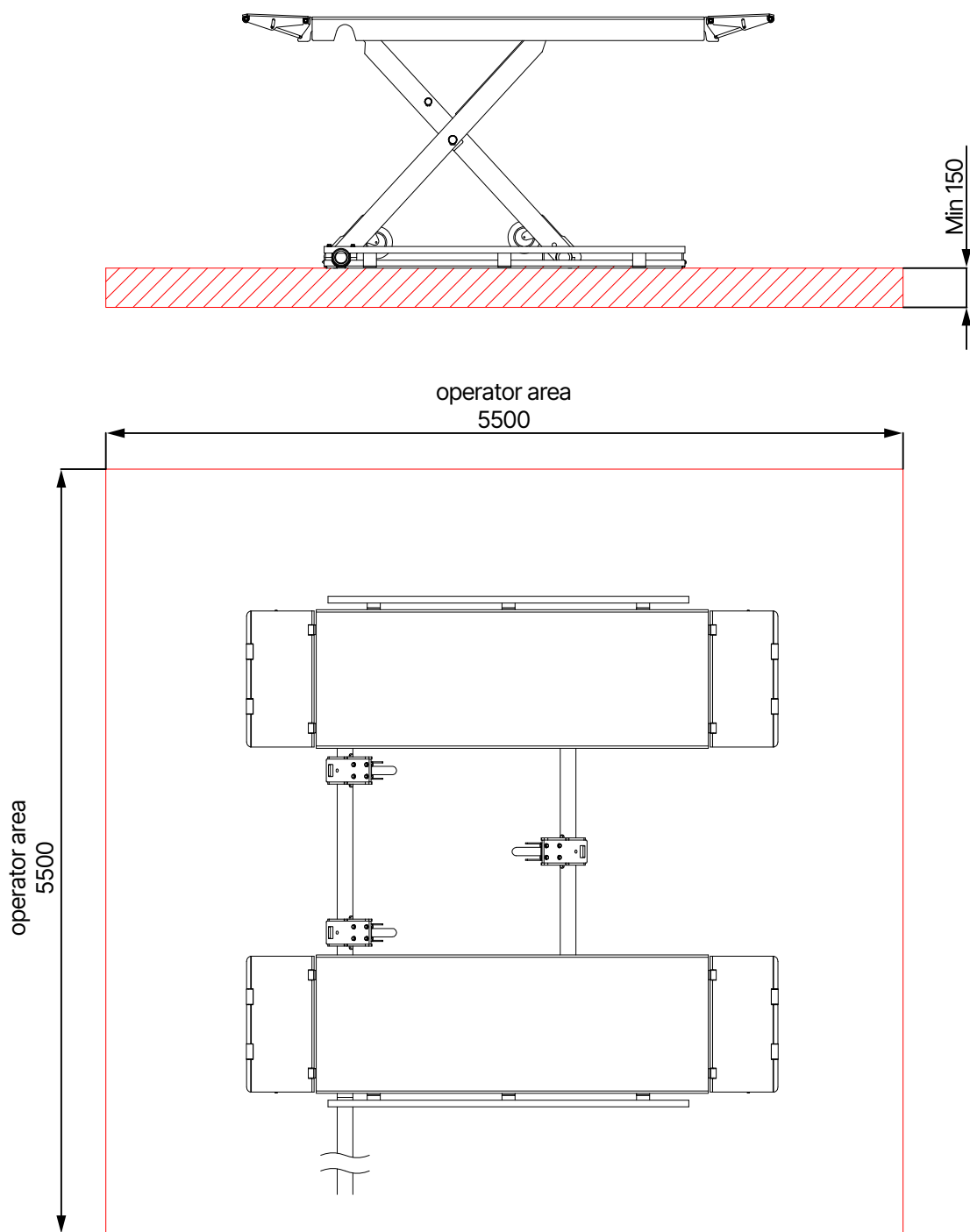
План фундаменту над землею
